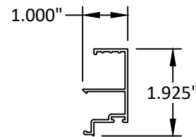
84 DOOR STOP
