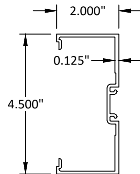
94 DOOR JAMB
