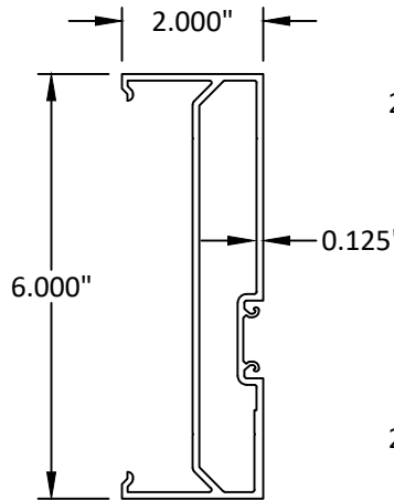
111 JAMB MULLION
