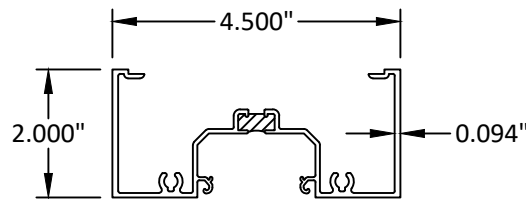
109 TRANSOM HEADER
