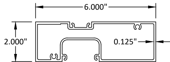
113 DOOR HEADER
