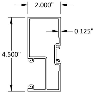
102 DOOR JAMB
