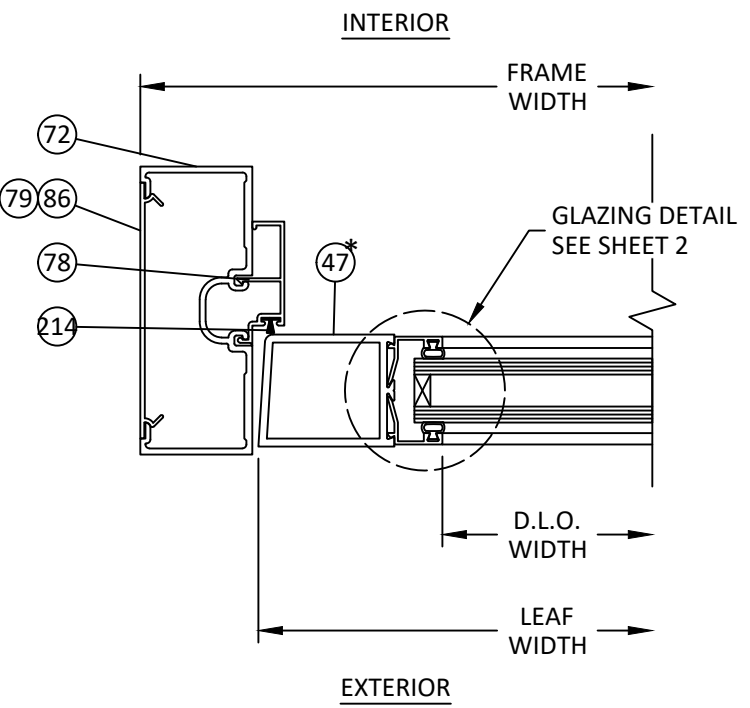
AF 14 HORIZONTAL SECTION DOOR JAMB FG-2000 FRAMING
