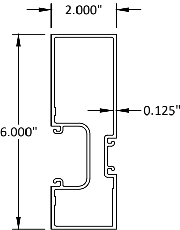
110 DOOR JAMB
