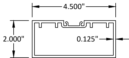
97 DOOR HEADER
