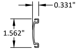
20 ASTRAGAL
