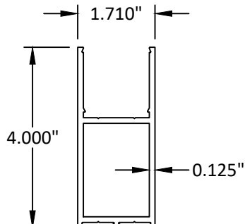
42 DOOR RAIL
