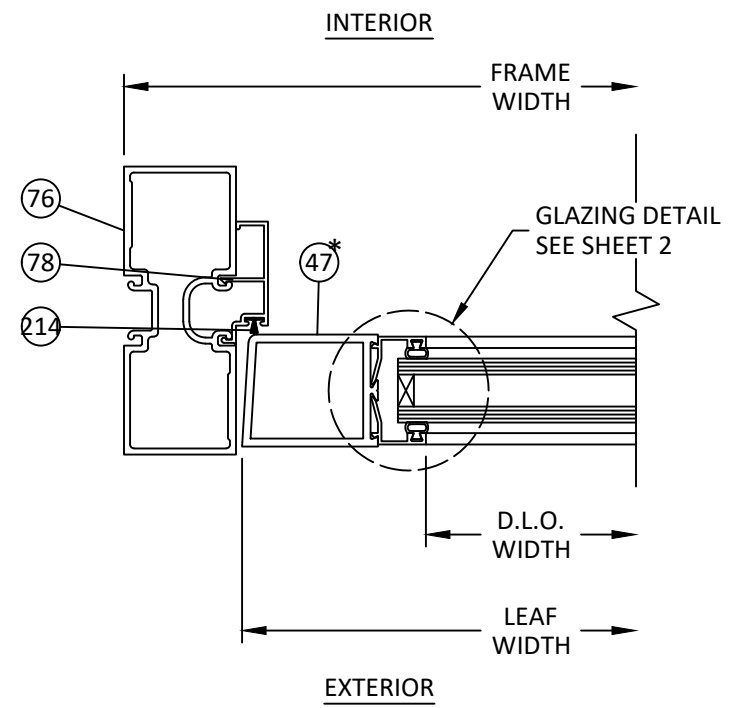
AG 14 HORIZONTAL SECTION DOOR JAMB FG-2000 FRAMING
