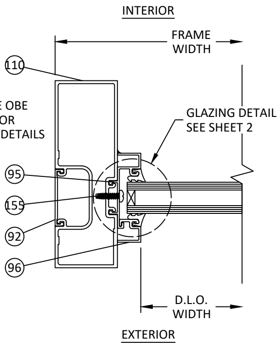
BL 18 HORIZONTAL SECTION TRANSOM JAMB 6000 MP FRAMING - CS
