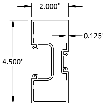
93 DOOR JAMB
