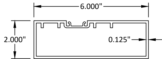
112 DOOR HEADER
